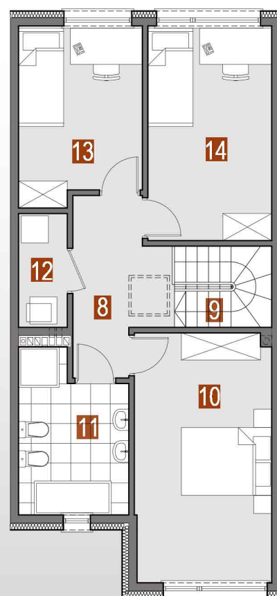
RZUT PIĘTRA
