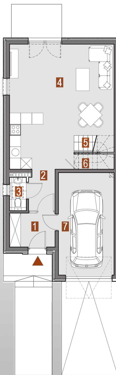
RZUT PARTERU
